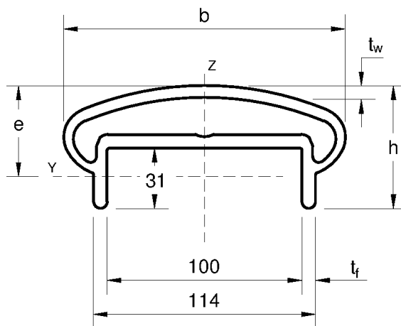
Handlauf 63 x 145
