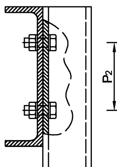
Schnitt C – C
