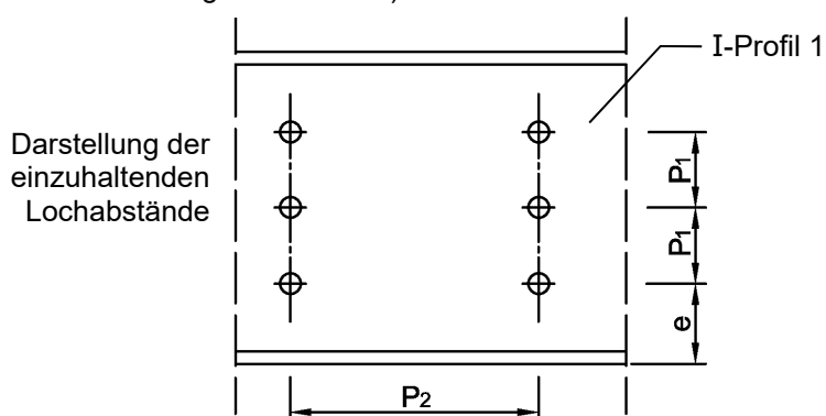
Ansicht B
