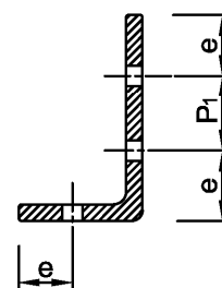
Schnitt B – B
